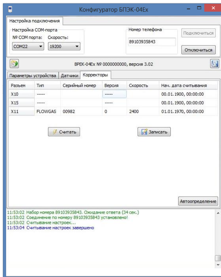
Рисунок 12 – Вкладка «Корректоры»
