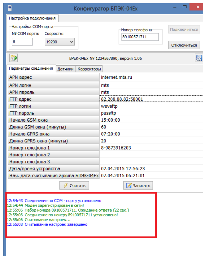
Рисунок 14 – протокол программы
